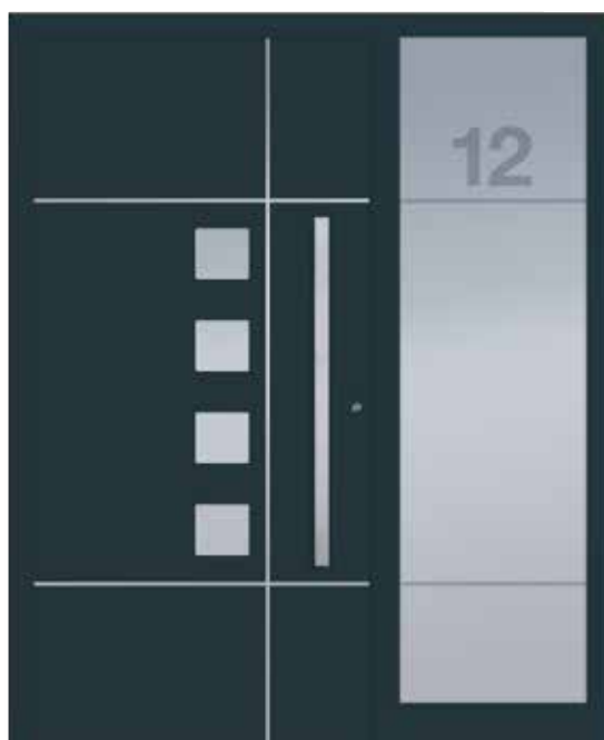
M-549 Ansicht A / DIN rechts Aufsatzfüllung Farbe Anthrazitgrau ähnl. RAL 7016 Feinstruktur flächenbündige Streifenapplikationen in Edelstahloptik außen Isolierglas Satinato weiß | GG 2 Griff ZAE 128, 1000 mm | PG 10 Seitenteil Sandstrahlmotiv ST 961 auf Klarglas individuelle Hausnummer
