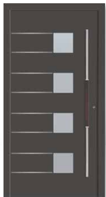
M-230 Ansicht A / DIN rechts Applikationen in Edelstahloptik außen und Rahmen in Edelstahloptik innen ■ Aufsatzfüllung ■ Farbe Eisenglimmer ähnl. DB 703 Feinstruktur ■ Isolierglas Satinato weiß | GG 2 ■ Griff ZAE 164, 1600 mm | PG 16 (Holzelement variabel einstellbar)
