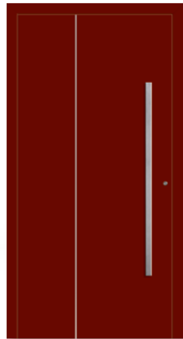
M-466 C aufgesetzte Streifenapplikation in Edelstahloptik außen ■ Aufsatzfüllung ■ Farbe Purpurrot ähnl. RAL 3004 Feinstruktur ■ Griff ZAE 147, 1200 mm | PG 11
