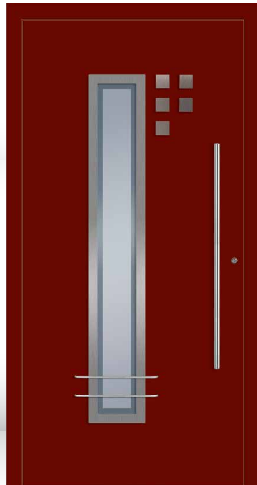
M-119 Ansicht B / DIN rechts Rahmen in Edelstahloptik beidseitig, Bügel und Applikationen in Edelstahloptik außen ■ Aufsatzfüllung ■ Farbe Purpurrot ähnl. RAL 3004 Feinstruktur ■ Sandstrahlmotiv Y 599 auf Klarglas | MG 1 ■ Griff ZAE 6, 1000 mm | PG 9
