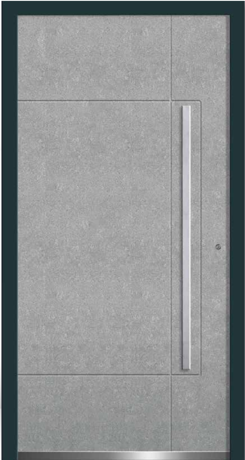
M-490 Ansicht A / DIN rechts Flachnuten außen ■ Aufsatzfüllung ■ Designoberfläche Concrete ■ Griff ZAE 147 | PG 11 ■ flächenbündiger Trittschutz TS 7
