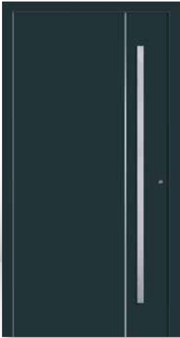
M-425 Ansicht A / DIN rechts ■ Aufsatzfüllung ■ Farbe Anthrazitgrau ähnl. RAL 7016 Feinstruktur ■ flächenbündige Streifenapplikation in Edelstahloptik außen ■ Griff ZAE 128, 1600 mm | PG 11
