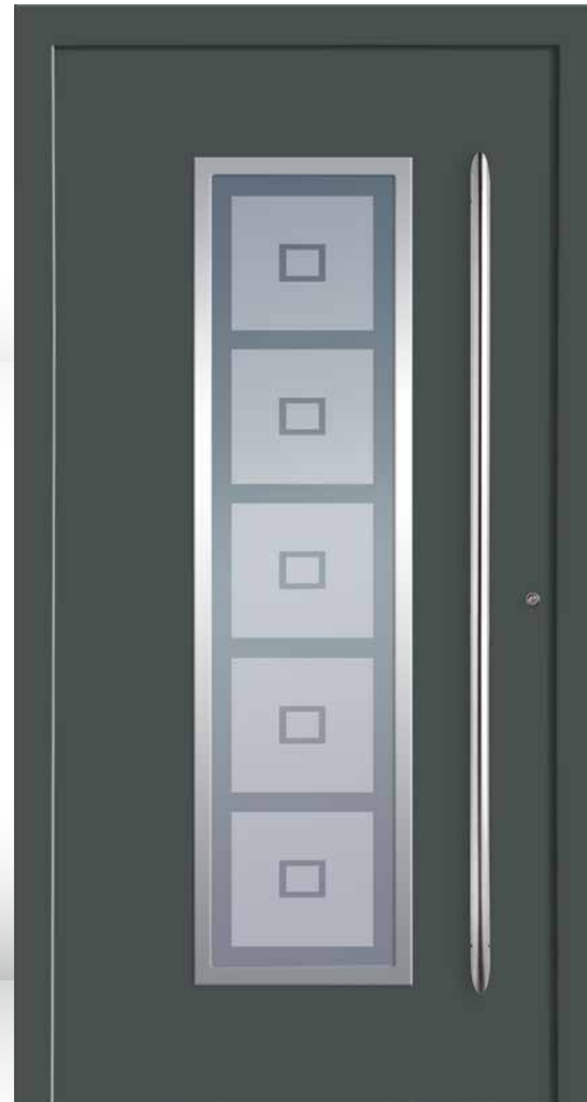
M-060 Rahmen in Edelstahloptik beidseitig ■ Aufsatzfüllung ■ Farbe Basaltgrau ähnl. RAL 7012 Feinstruktur ■ Sandstrahlmotiv Y 922 auf Klarglas | MG 1 ■ Griff ZAE 107, 1585 mm | PG 11
